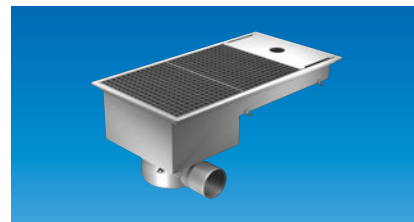
STÅDRUMSBRUNN FURO 325: Rostfri kvalitet EN 1.4301, sido- eller bottenutlopp, storlek 600 x 400 mm.
