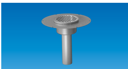
GJUTASFALTBRUNN FURO 184, 185: Syrafast kvalitet EN 1.4404, bottenutlopp.
